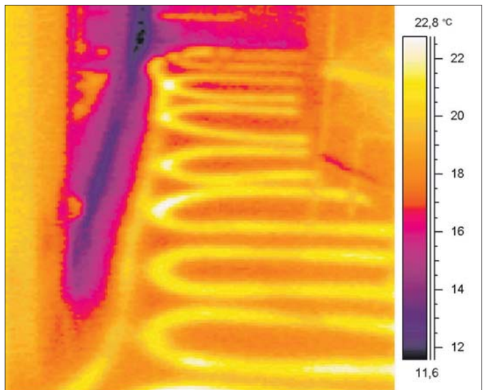
Mit einer Wärmebildkamera erkennen die Experten der Firma Freund, wie eine Fußbodenheizung verteilt ist und wo zum Beispiel Kältebrücken sind. So kann das Heizungssystem optimal eingestellt werden.
