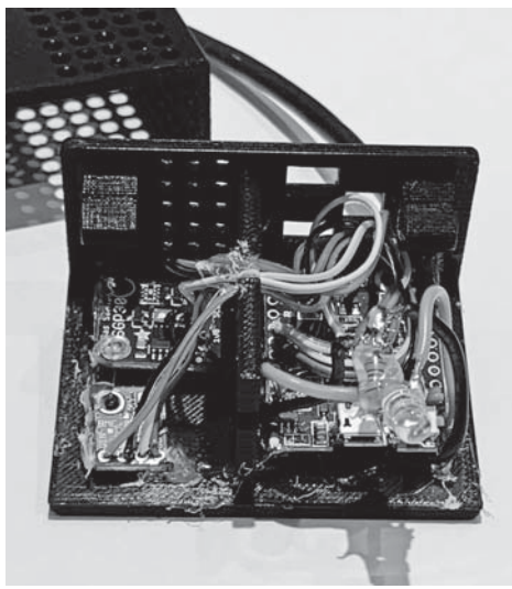
Recht kompliziert sieht es im inneren der Messgeräte aus. Foto: AES
